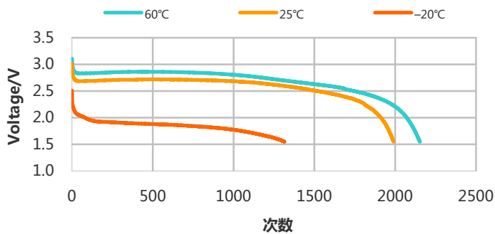
不同温度放电曲线 ( 0.9A 3sec.on/27sec.off )
