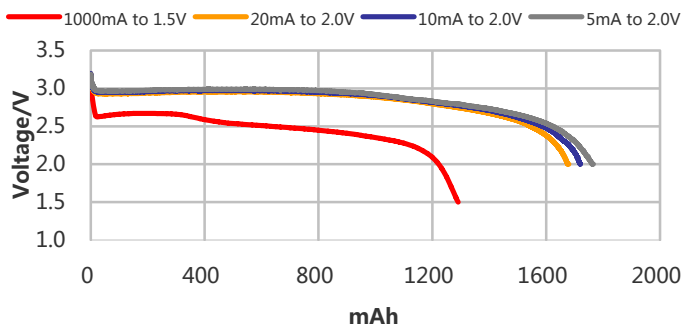
不同电流放电曲线 ( 25°C )
